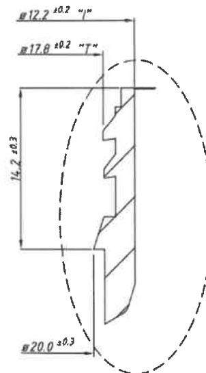
DETALHE A ESCALA 3:1
